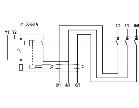
DS 203
