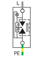
OVR T1 25 255-7
