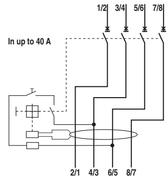
DS 204
