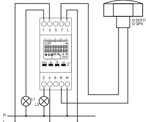
D2 SYNCHRO
