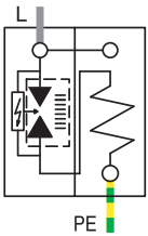
OVR T1 25 255
