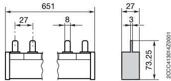
S800-BB250
