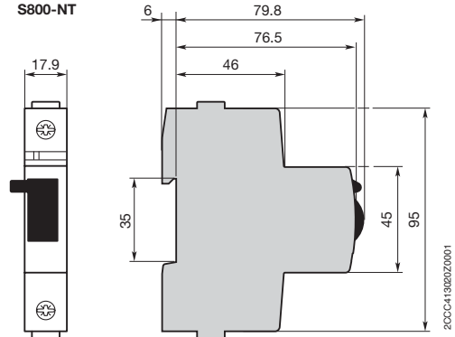
S800-NT
