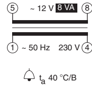
TS8/12 SW
