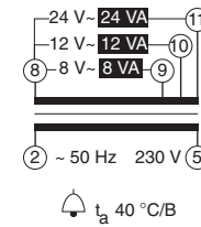
TS24/8-12-24
