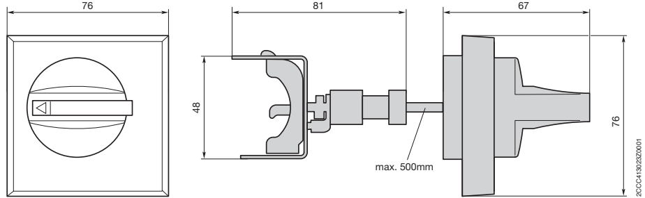
S800-RD+S800-RHE
