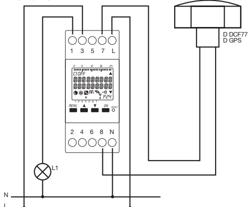
D1 SYNCHRO
